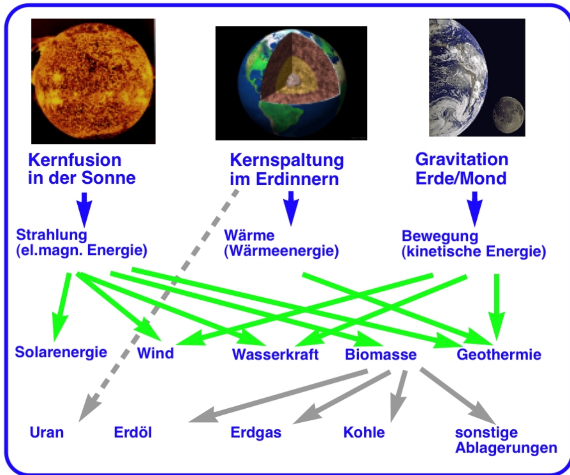
Bild 1.2: Nutzbares Energiespektrum
