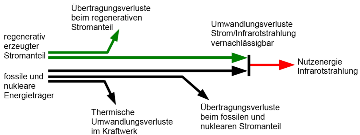
Bild 3.4: Energiefluss der Infrarotheizung
