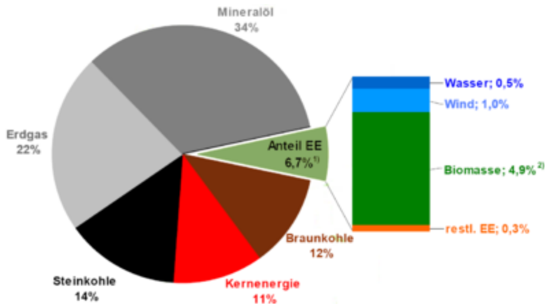
Bild 1.3: Primärenergieverbrauch Deutschland
