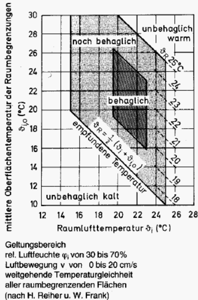
Bild 1.7: Strahlungstemperatur-Lufttemperatur-Diagramm
